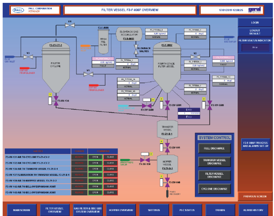
Esquema de la pantalla de control del PLC.
